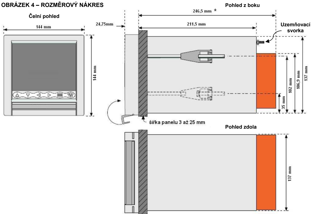
OBRÁZEK 4 – ROZMĚROVÝ NÁKRES
