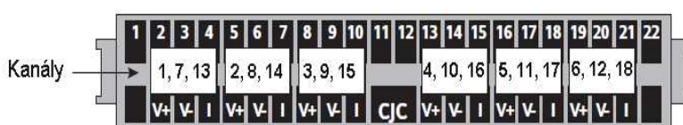
OBRÁZEK 6 - ZAPOJENÍ VSTUPNÍCH KANÁLŮ
