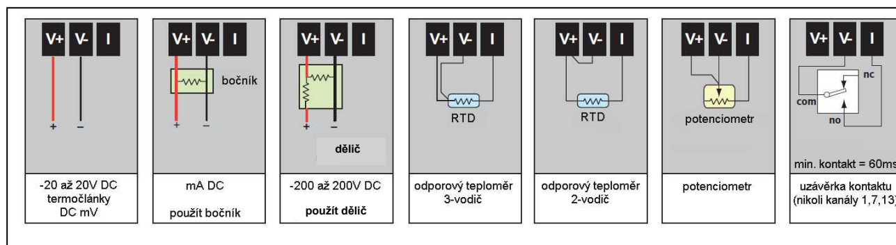
OBRÁZEK 7: ZAPOJENÍ VSTUPNÍCH SIGNÁLŮ
