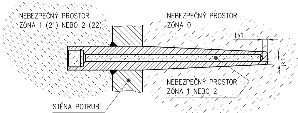
OBRÁZEK 2 – JÍMKA PRO SNÍMAČ TEPLoty Ex d PRO ZÓNU 0 (dle ČSN EN 60079-26 ed.2)
