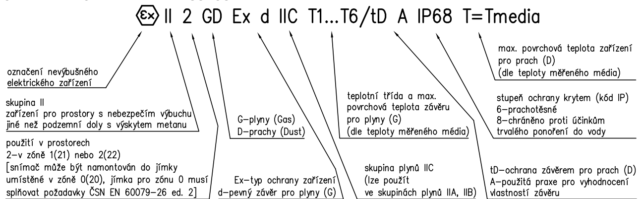
OBRÁZEK 1 - OZNAČENÍ NEVÝBUŠNOSTI
