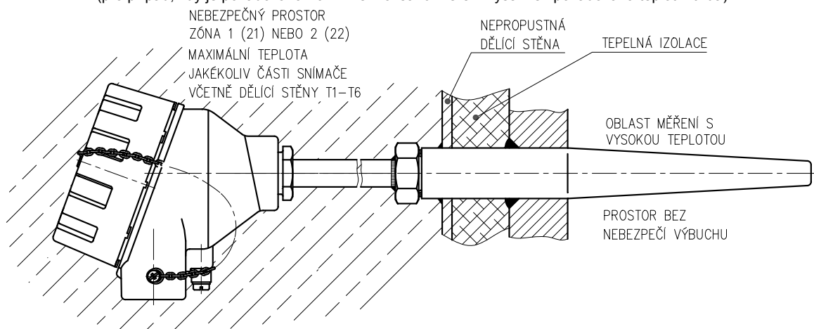
OBRÁZEK 3 - PŘÍKLAD MONTÁŽE SNÍMAČŮ TEPLoty Ex d DO JÍMKY DIN
