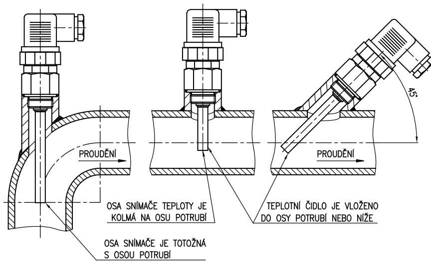
OBRÁZEK 3 - PŘÍKLADY MONTÁŽE PŘÍMÝCH A ŠIKMÝCH NÁVARKŮ DLE ČSN EN 1434-2
