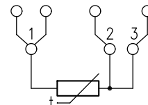
SCHÉMA ZAPOJENÍ KONEKTORU SNÍMAČE JAKO ČTYŘVODIČ:
