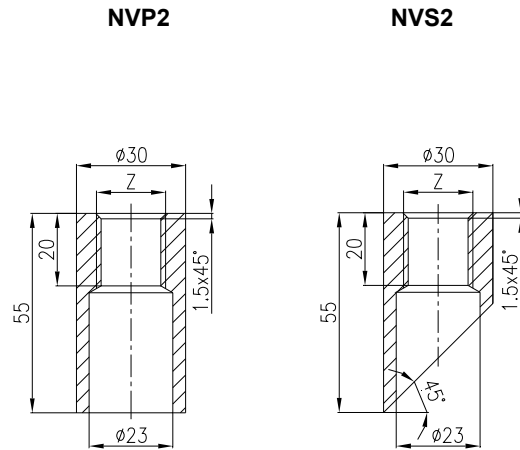
OBRÁZEK 2 - ROZMĚROVÝ NÁKRES NÁVARKŮ
