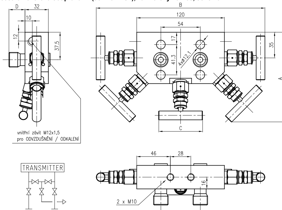
Obrázek 10 - Pěticestná ventilová souprava (964 25.. AS2), rozměrový nákres, schéma
