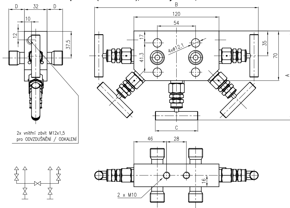
Obrázek 15 - Pěticestná ventilová souprava (964 45.. AS1), rozměrový náčrtek, schéma
