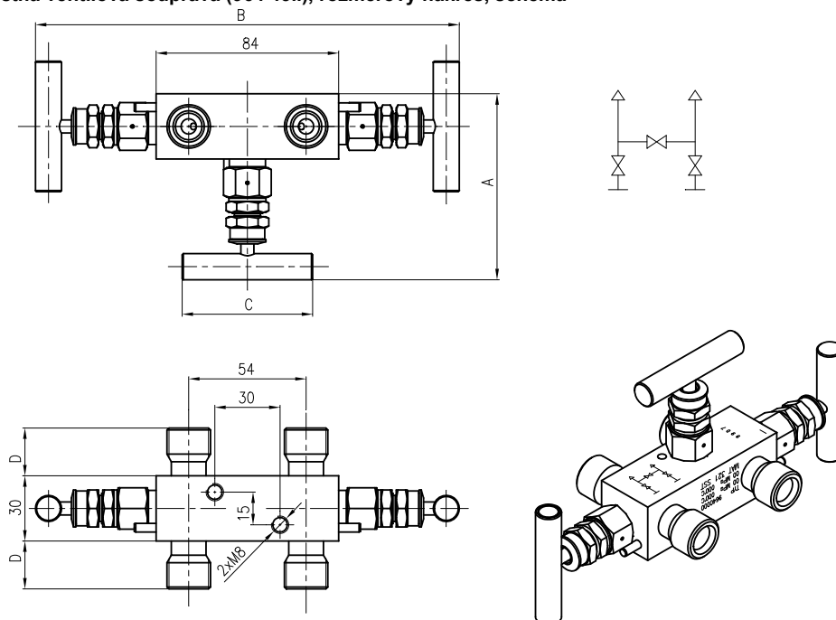
Obrázek 5 - Třicečná ventilová souprava (964 43..), rozměrový nákres, schéma
