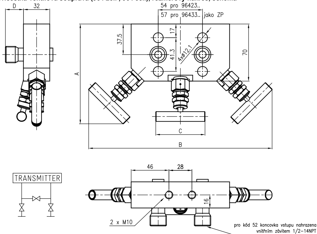
Obrázek 4 - Třícestná ventilová souprava (964 23.. , 964 33..), rozměrový náčrtek, schéma
