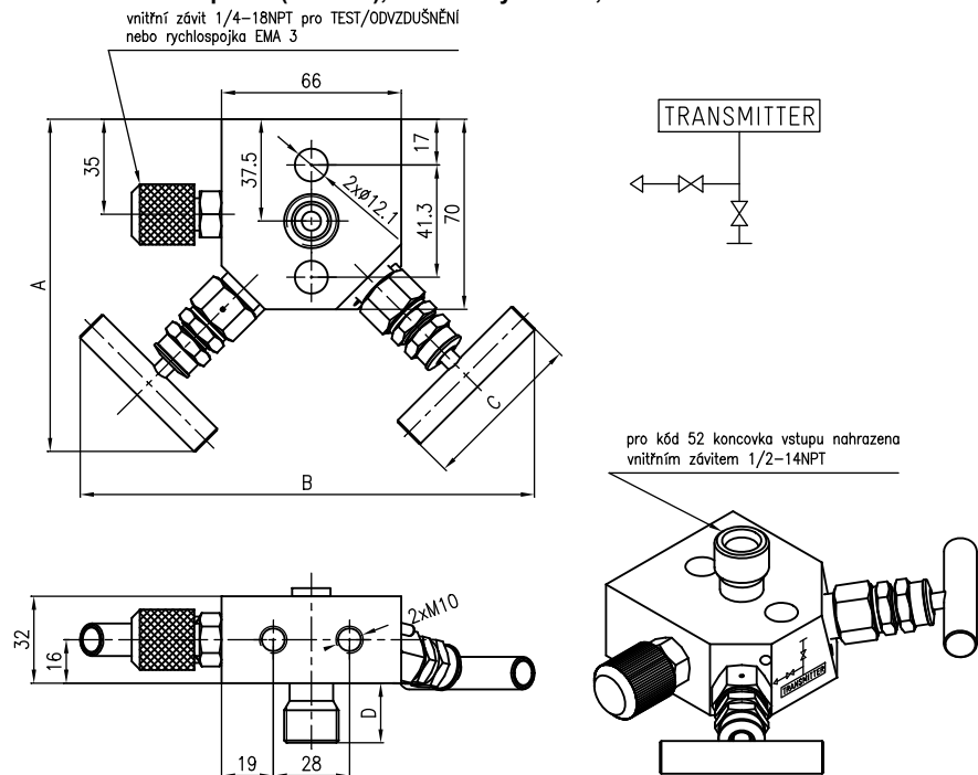
Obrázek 1 - Dvoucestná ventilová souprava (964 21..), rozměrový náčrtek, schéma
