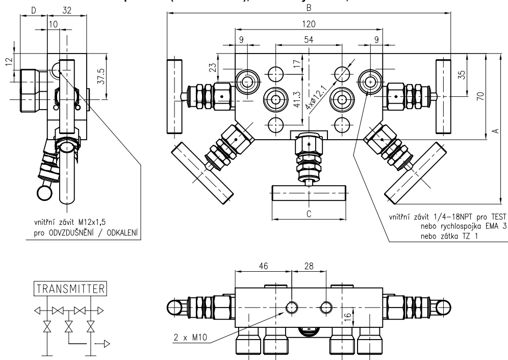
Obrázek 13 - Pěticestná ventilová souprava (964 25.. AS21), rozměrový nákres, schéma
