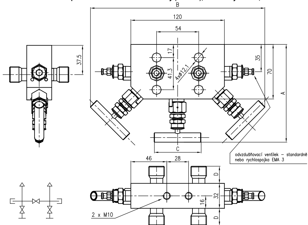
Obrázek 7 - Třicečná ventilová souprava s odvzdušňovacími ventilkami (964 44..), rozměrový nákres, schéma
