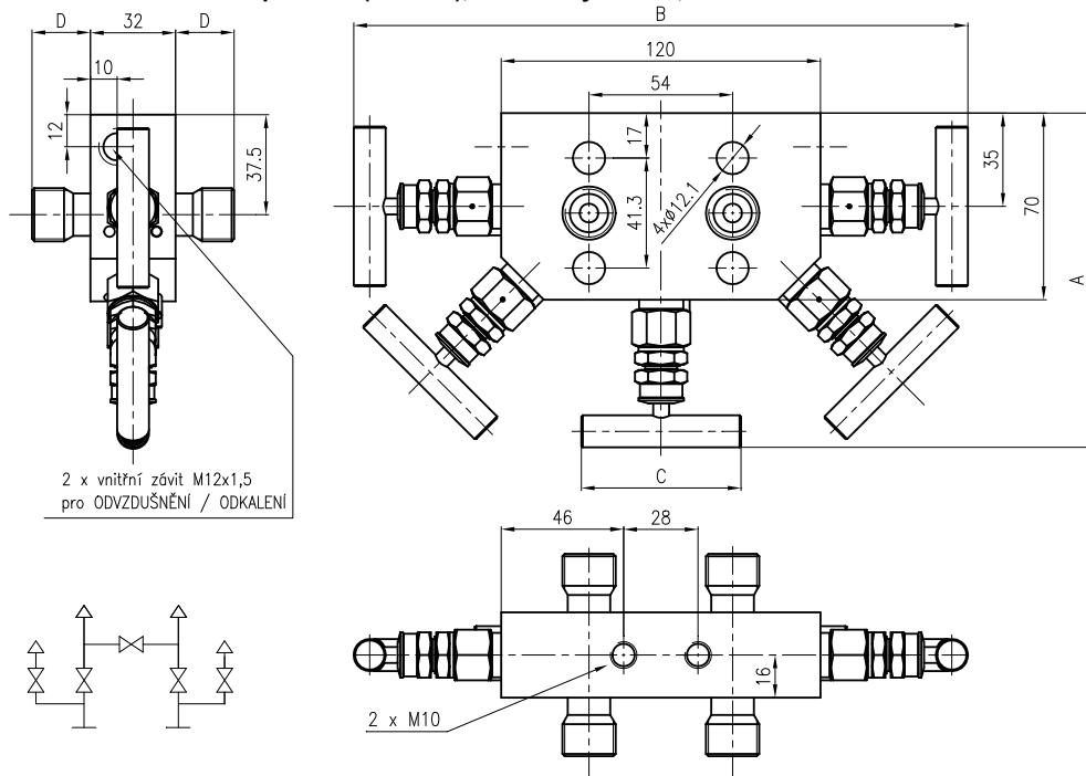
Obrázek 14 - Pěticestná ventilová souprava (964 45..), rozměrový nákres, schéma
