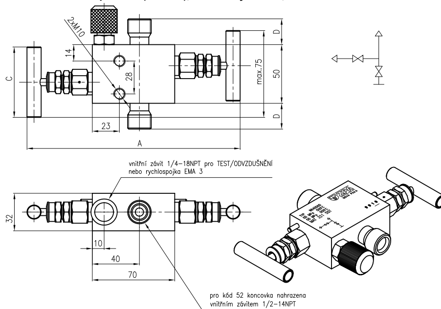
Obrázek 3 - Dvoucestná ventilová souprava (964 41..), rozměrový náčrtek, schéma
