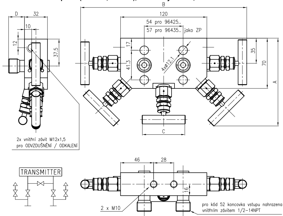
Obrázek 8 - Pěticečná ventilová souprava (964 25.. , 964 35..), rozměrový nákres, schéma
