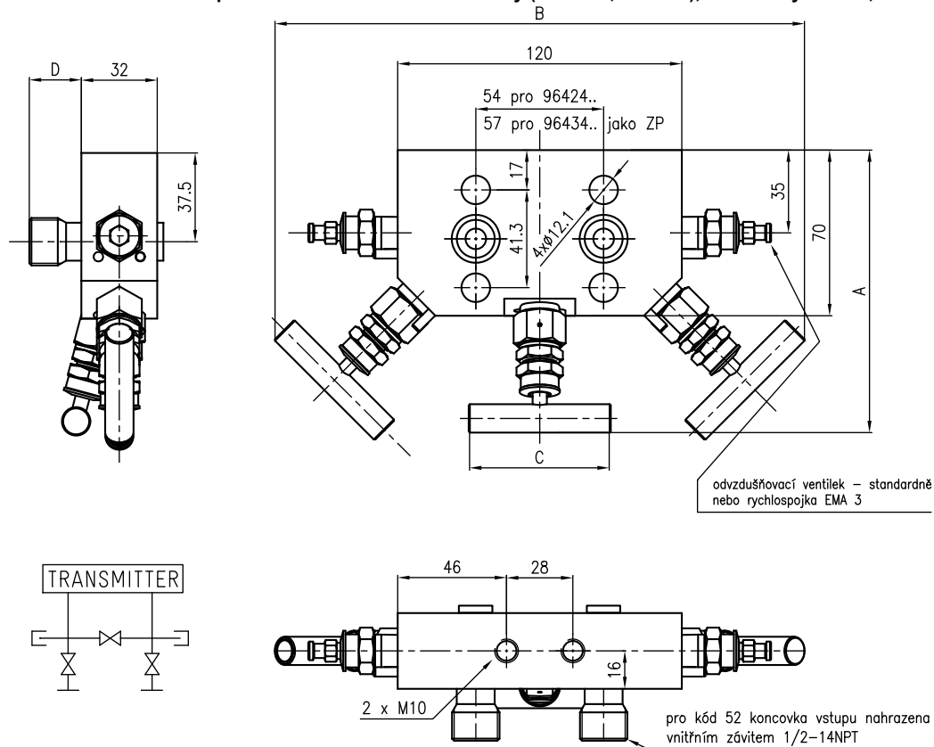
Obrázek 6 - Třicečná ventilová souprava s odvzdušňovacími ventilkou (964 24.. , 964 34..), rozměrový nákres, schéma
