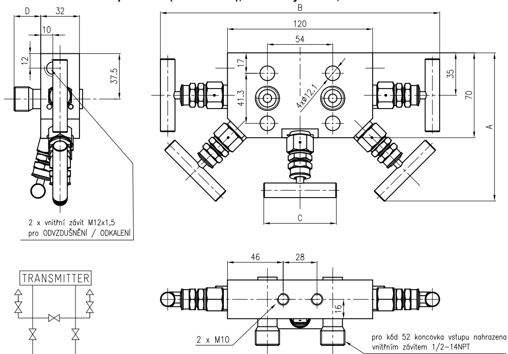
Obrázek 9 - Pěticestná ventilová souprava (964 25.. AS1), rozměrový nákres, schéma
