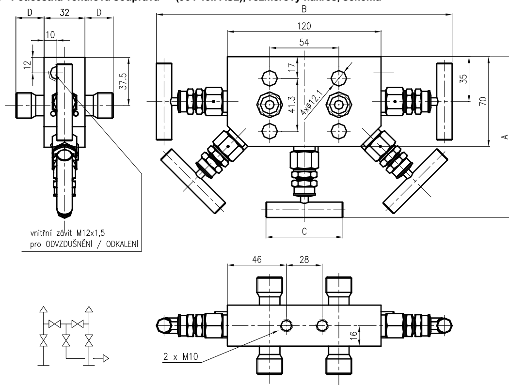
Obrázek 16 - Pěticestná ventilová souprava (964 45.. AS2), rozměrový náčrtek, schéma
