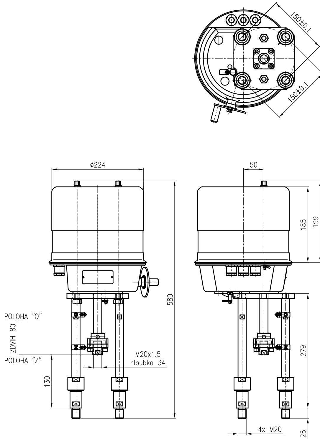
OBRAZEK 3 ROZMĚROVÝ NÁKRES - PŘIPOJENÍ P5 - ROZTEČ 150, 4 SLOUPKY M20, SPOJKA M20X1,5, ZDVIH 80
