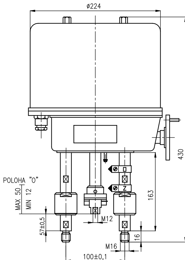
OBRÁZEK 1 - ROZMĚROVÝ NÁKRES – PŘIPOJENÍ P2
