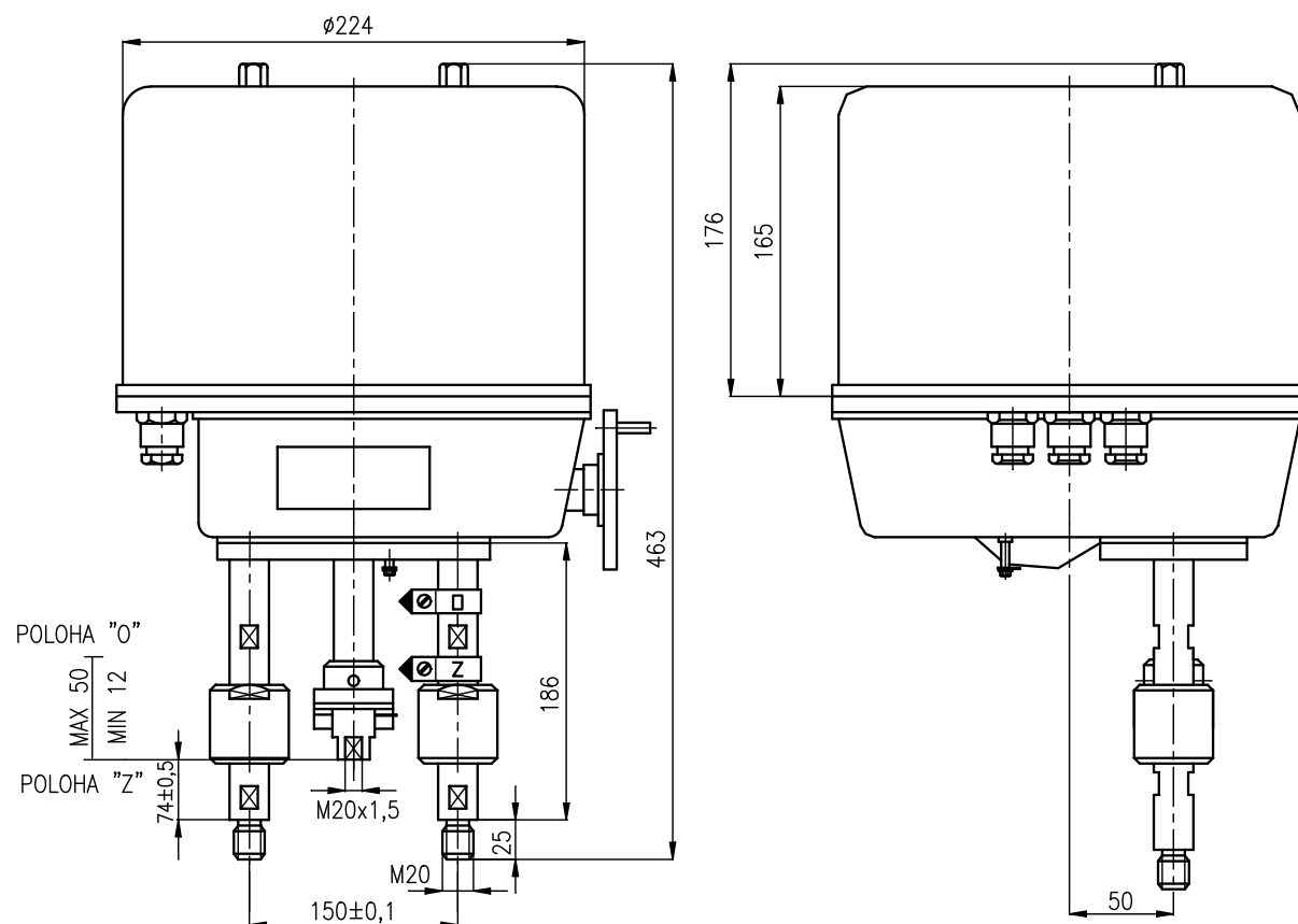
OBRÁZEK 5 - ROZMĚROVÝ NÁKRES – PŘIPOJENÍ P8
